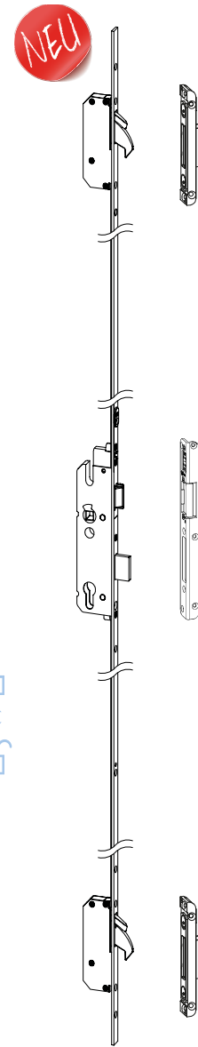
AV4D Automatik Verriegelung mit Tagesfallen Funktion 3 - fach mit 2 Haken , Farbe Topzink Tag / Nacht Funktion - für temporär flexibles Ein- und Austreten ohne Schlüsseldrehung
